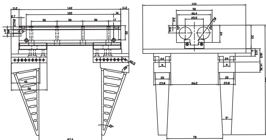
固定座可調整距離 Fixed seat adjustable distance
