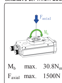
模組出力表Pinion Load
