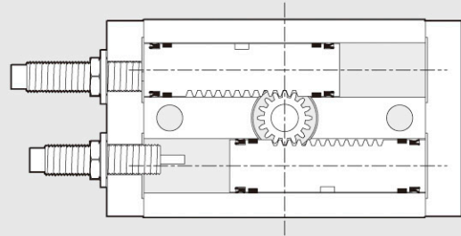
內部結構圖 Internal structure
