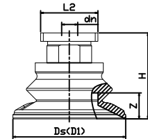
VAF-1.5 30 至 100 RA(矩形適配器)
