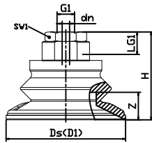
VAF-1.5 30 至 100 IH
