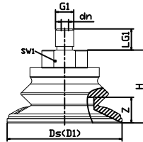
VAF-1.5 30 至 100 EH
